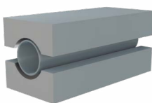
7 Окончательная формовка трубной заготовки
